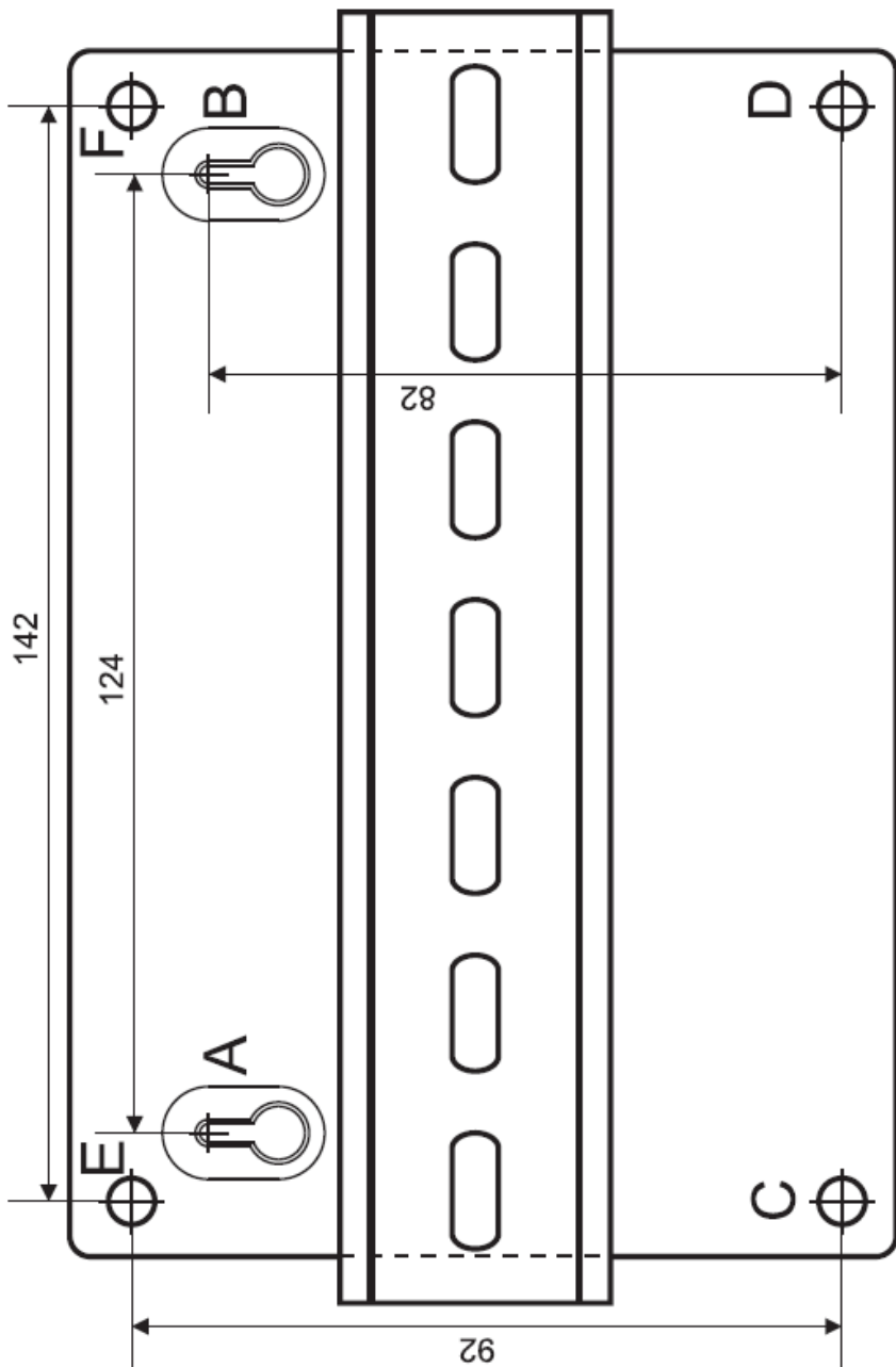
Рисунок 20. Шаблон для монтажа
